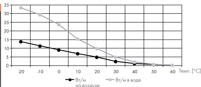
Выходная мощность при данной температуре (вода/воздух)
